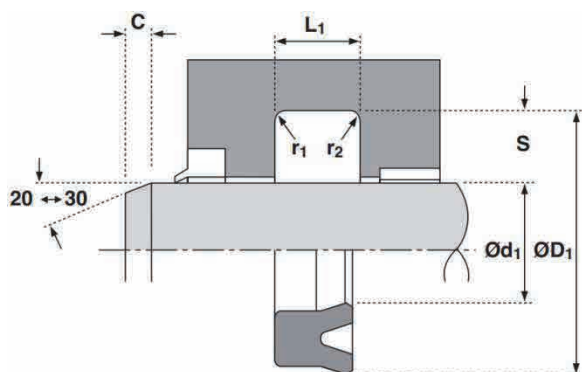
Rod Seal
